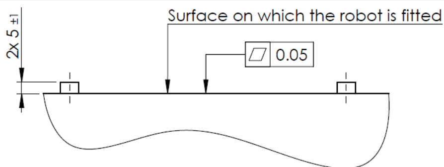
1.2: Montážní deska pro základnu robota
