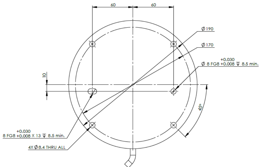
1.1: Pohled na základnu robota zespodu
